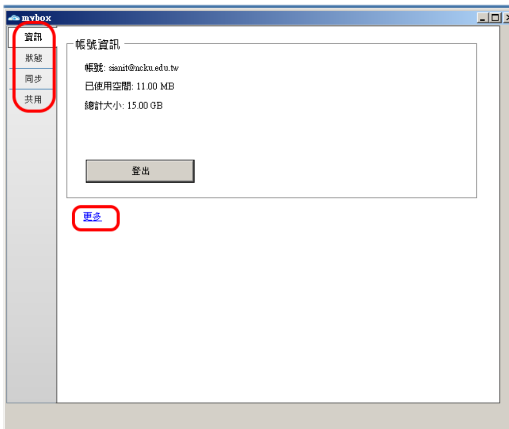
圖 8：Windows 版 mybox 功能標籤頁：資訊
